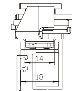
C groove friction hinge FH06
