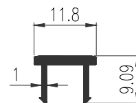
42792 WT : 0.093 Kg./m. ตบรางหัวแบน
