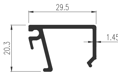
30055 (GL 6mm.) WT : 0.315 Kg./m. คิ้วบานเปิดร่อง 12.7 มม.
