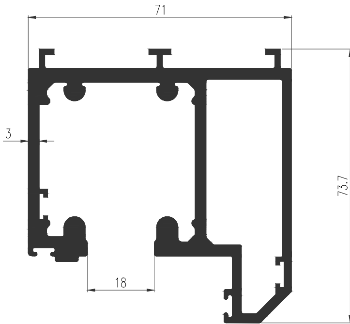
30063 WT : 2.961 Kg./m. เฟรมบานบานพิเศษ
