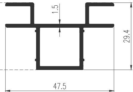
42111 WT : 0.574 Kg./m. ตัวต่อราง
