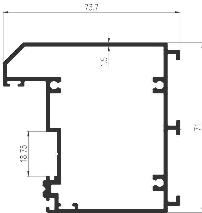
30263 WT : 1.459 Kg./m. เฟรมข้างบานพิเศษ
