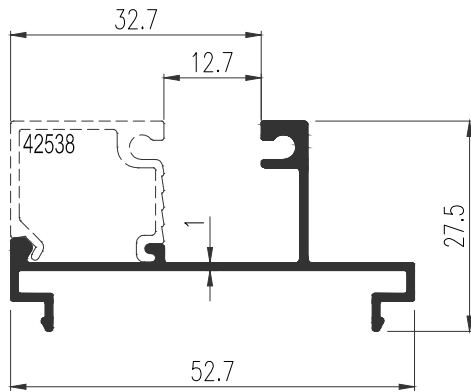
42539 WT : 0.349 Kg./m. ตบช่องแสง (52.7 มม.)
