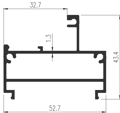
42537 WT : 0.737 Kg./m. วงกบช่องแสง (52.7 มม.)
