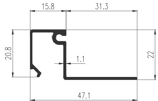
50726 (GL 24mm.) WT : 0.292 Kg./m. คิ้วช่องแสงร่อง 29.5 มม.
