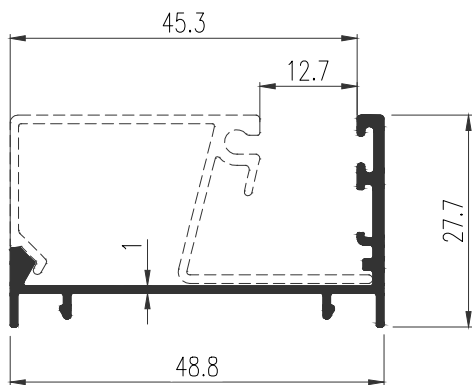
50611 WT : 0.329 Kg./m. ตบช่องแสง (48.8 มม.)
