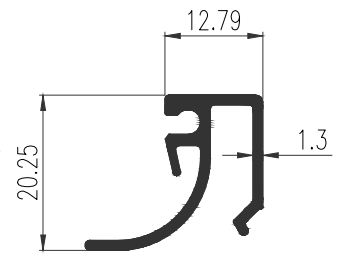
30265 (GL 24mm.) WT : 0.253 Kg./m. คิ้วบานเปิดร่อง 29.4 มม.
