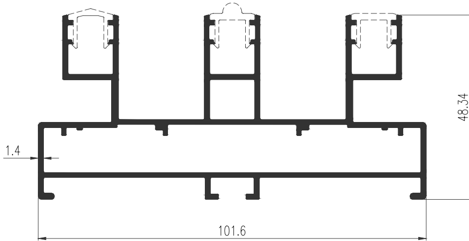
42787 WT : 1.701 Kg./m. เฟรม 3 ราง เปิดหัว (101.6 มม.)
