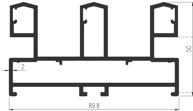
42836 WT : 2.343 Kg./m. เฟรม 3 ราง (89.8 มม.)
