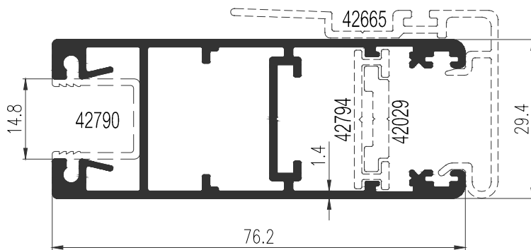
42664 WT : 1.157 Kg./m. กรอบบาน 3 นิ้ว ร่อง 14.8 มม.
