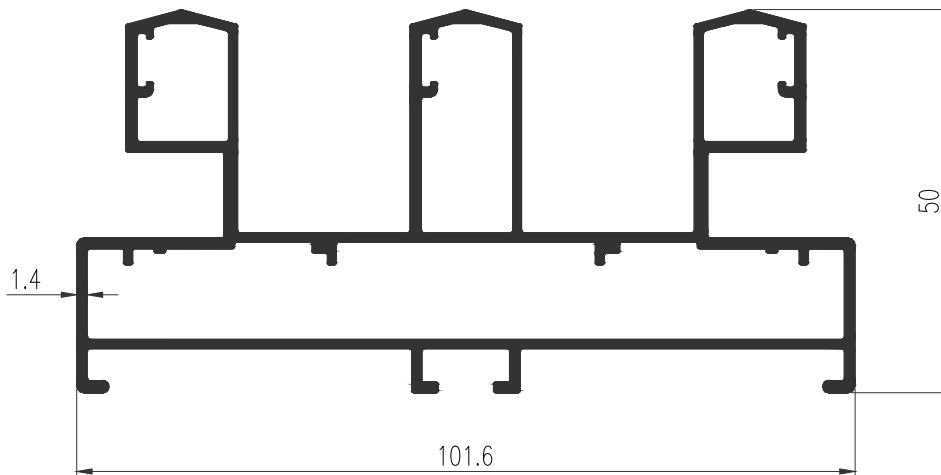
42778 WT : 1.783 Kg./m. เฟรม 3 ราง (101.6 มม.)
