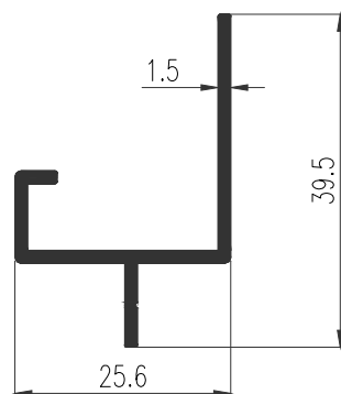
42562 WT : 0.308 Kg./m. เฟรมรับพื้น
