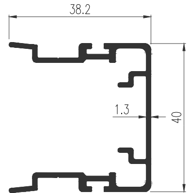
42446 WT : 0.573 Kg./m. ตบเกี้ยวสองทาง
