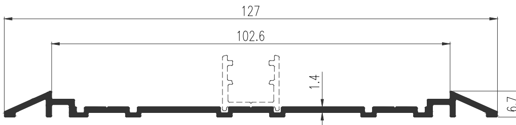
43158 WT : 0.584 Kg./m. รางล่างบานเลื่อนภายใน
