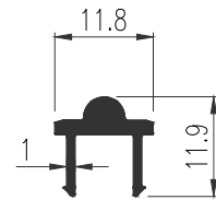
42311 WT : 0.125 Kg./m. ตบรางหัวกลม
