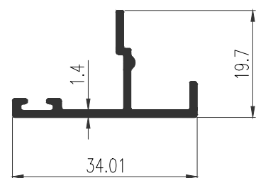
30066 WT : 0.246 Kg./m. บังใบบานพิเศษ
