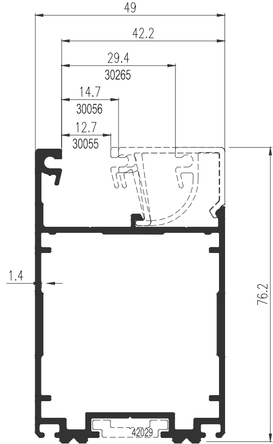
30508 WT : 1.230 Kg./m. กรอบบานเฟี้ยมแกนสไลด์
