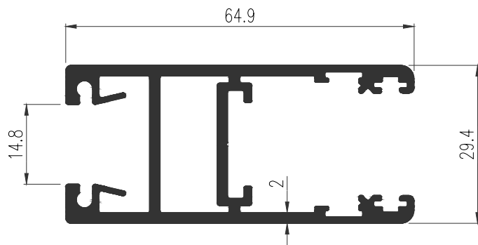
42835 WT : 1.247 Kg./m. กรอบบานร่อง 14.8 มม.
