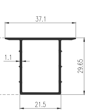
42789 WT : 0.339 Kg./m. ตบปิดราง
