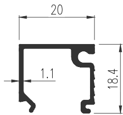
42538 (GL 6mm.) WT : 0.207 Kg./m. คิ้วช่องแสง
