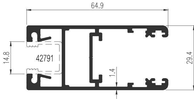
42026 WT : 1.044 Kg./m. กรอบบานร่อง 14.8 มม.
