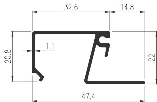
50612 (GL 6mm.) WT : 0.350 Kg./m. คิ้วช่องแสงร่อง 12.7 มม.
