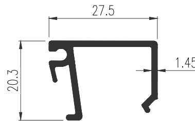
30056 (GL 8mm.) WT : 0.304 Kg./m. คิ้วบานเปิดร่อง 14.7 มม.
