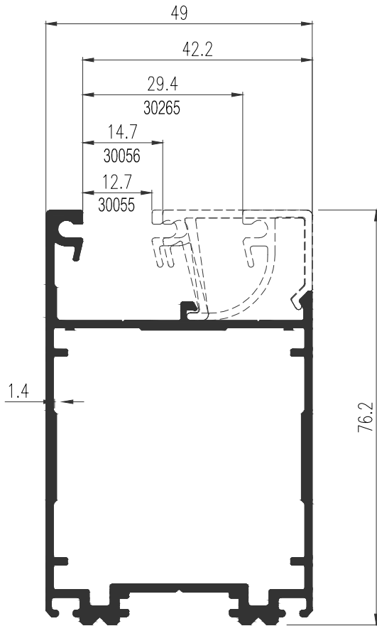
30264 WT : 1.242 Kg./m. กรอบบานเฟี้ยม
