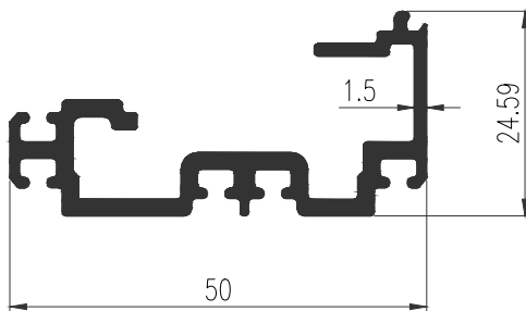
30061 WT : 0.678 Kg./m. ชนกลางบานเฟี้ยม
