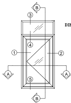
ELEVATION
