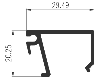
30055 (GL 6mm.) WT : 0.315 Kg./m. คิ้วบานเปิดร่อง 12.7 มม.
