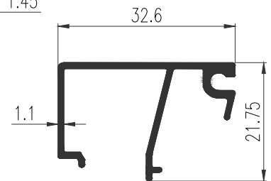
50753 (GL 6mm.) WT : 0.287 Kg./m. คิ้วช่องแสงร่อง Groove
