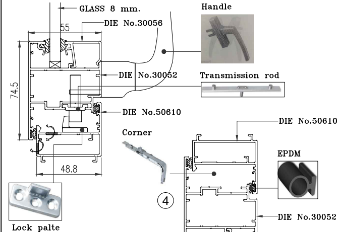
Lock palte
