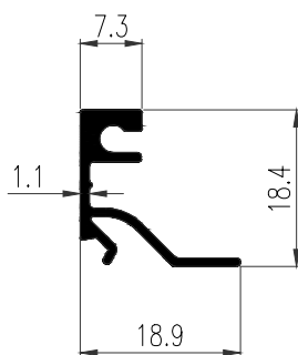
43221 (GL 20mm.) WT : 0.183 Kg./m. คิ้วตบช่องแสง 25.4 มม.
