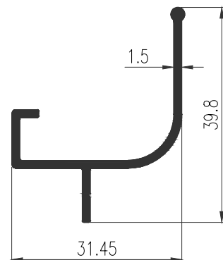
42109 WT : 0.322 Kg./m. หมวกหลบน้ำ
