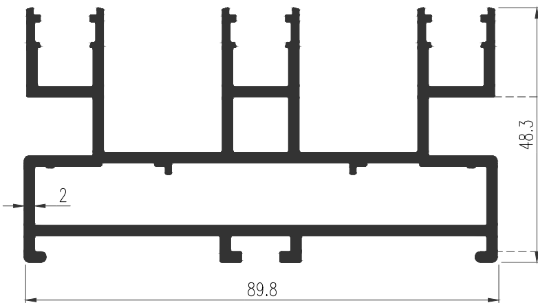
42837 WT : 2.197 Kg./m. เฟรม 3 ราง หัวเปิด (89.8 มม.)
