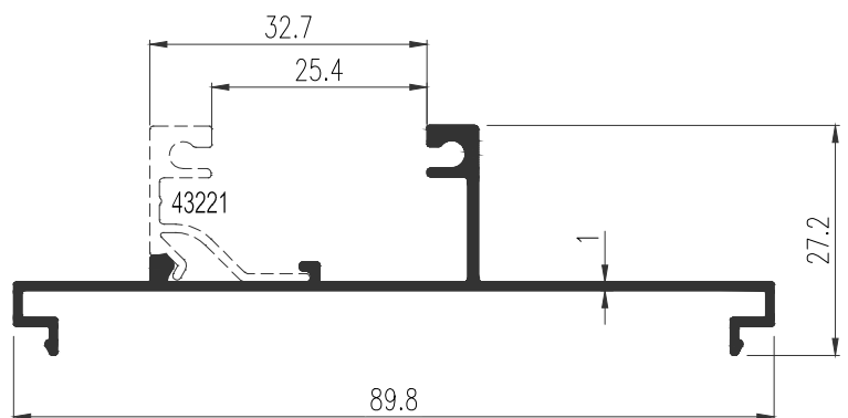
42560 WT : 0.452 Kg./m. ตบช่องแสง (89.8 มม.)
