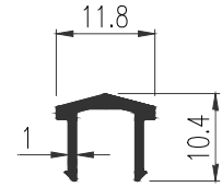
42310 WT : 0.090 Kg./m. ตบรางหัวเหลี่ยม
