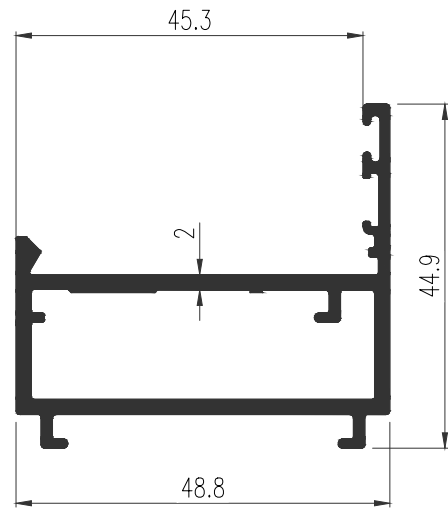
50675 WT : 0.924 Kg./m. เฟรมบานกระทุ้ง (48.8 มม.)
