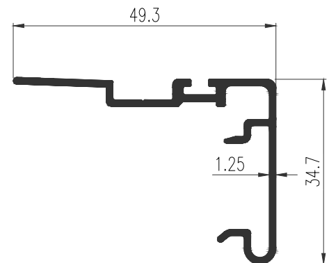
42665 WT : 0.422 Kg./m. ตบเกี้ยวบาน 3 นิ้ว
