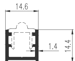
43159 WT : 0.156 Kg./m. รางบานเลื่อนตัวยู
