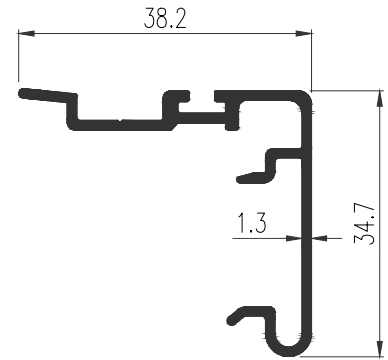
42028 WT : 0.382 Kg./m. ตบเกี้ยว
