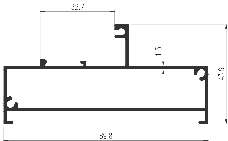
42559 WT : 0.998 Kg./m. วงกบช่องแสง (89.8 มม.)
